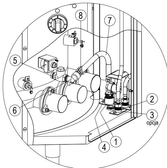
Rysunek 4a – Instalacja automatycznego napełniania ogrzewacza
