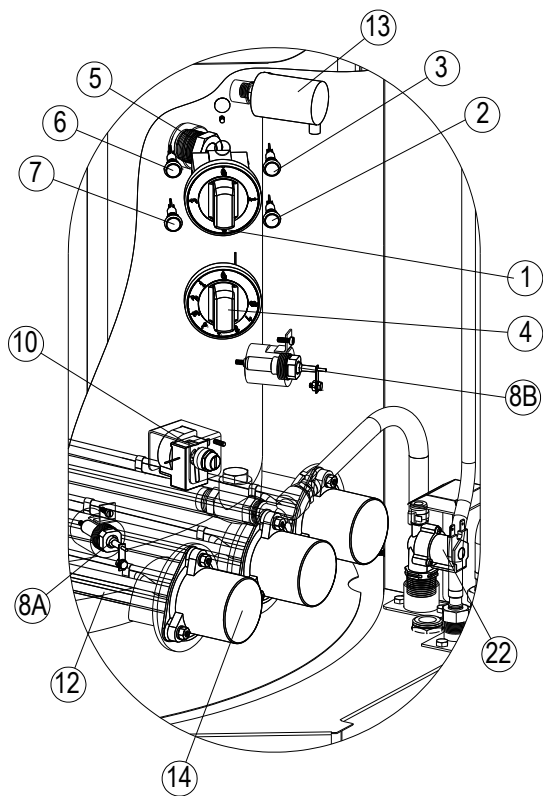
Ogranicznik temperatury poz. 10 Czujnik regulatora temperatury poz. 5
